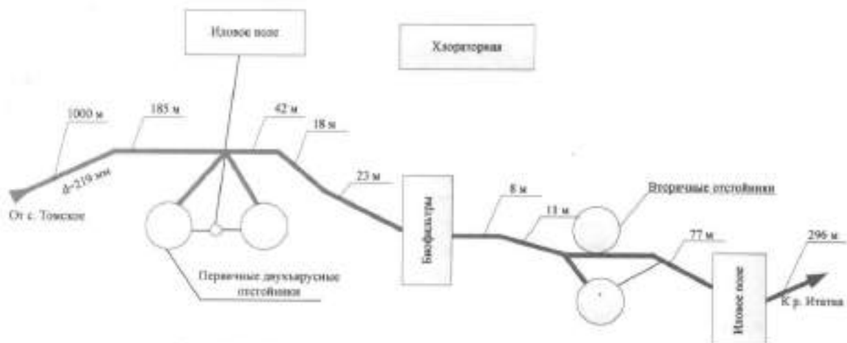
Рис. 1.5. Схема системы очистки и сброса сточных вод
