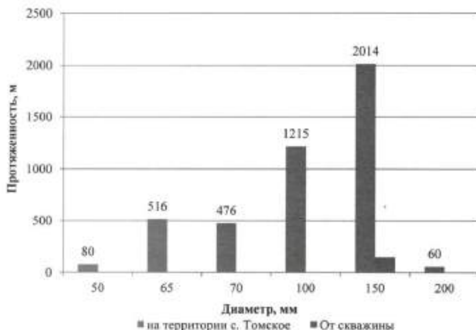
Рис. 1.3. Структура водопроводных сетей с. Томское
